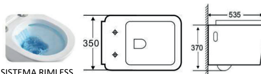
SISTEMA RIMLESS
