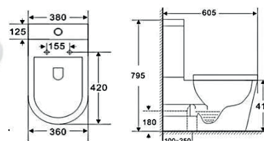
SISTEMA RIMLESS
